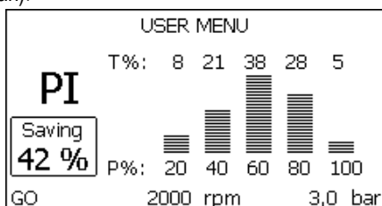
Kuva 17.1: Tehohistogrammin näyttö (1)
