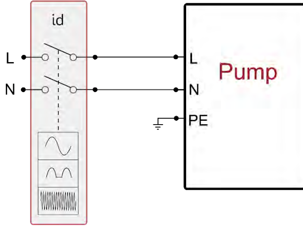
Şekil 10 Montaj Örneği
